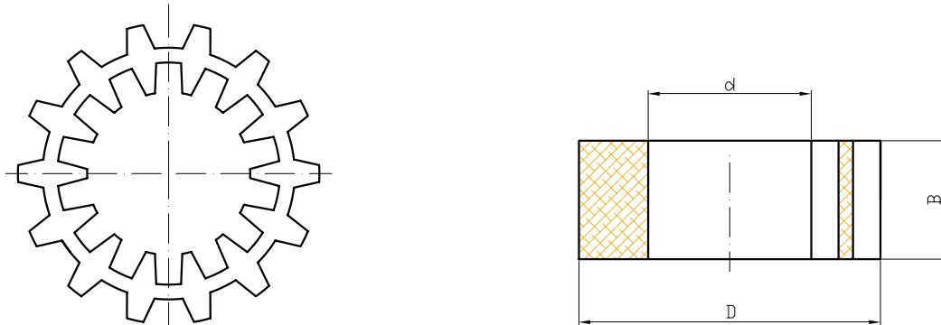
Zahnring Elastomer flexibels
