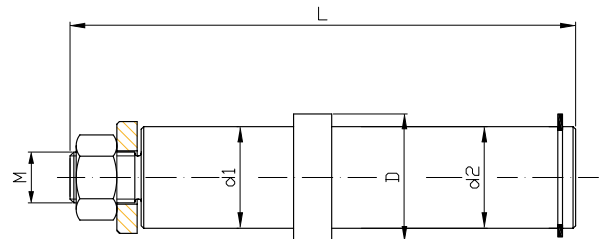
Größe 018 – 065 Size 018 – 065
