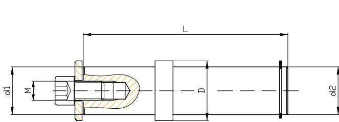
Größe 009 – 015 Size 009 – 015
