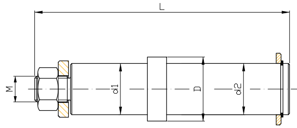
Größe 100 – 140 Size 100 – 140
